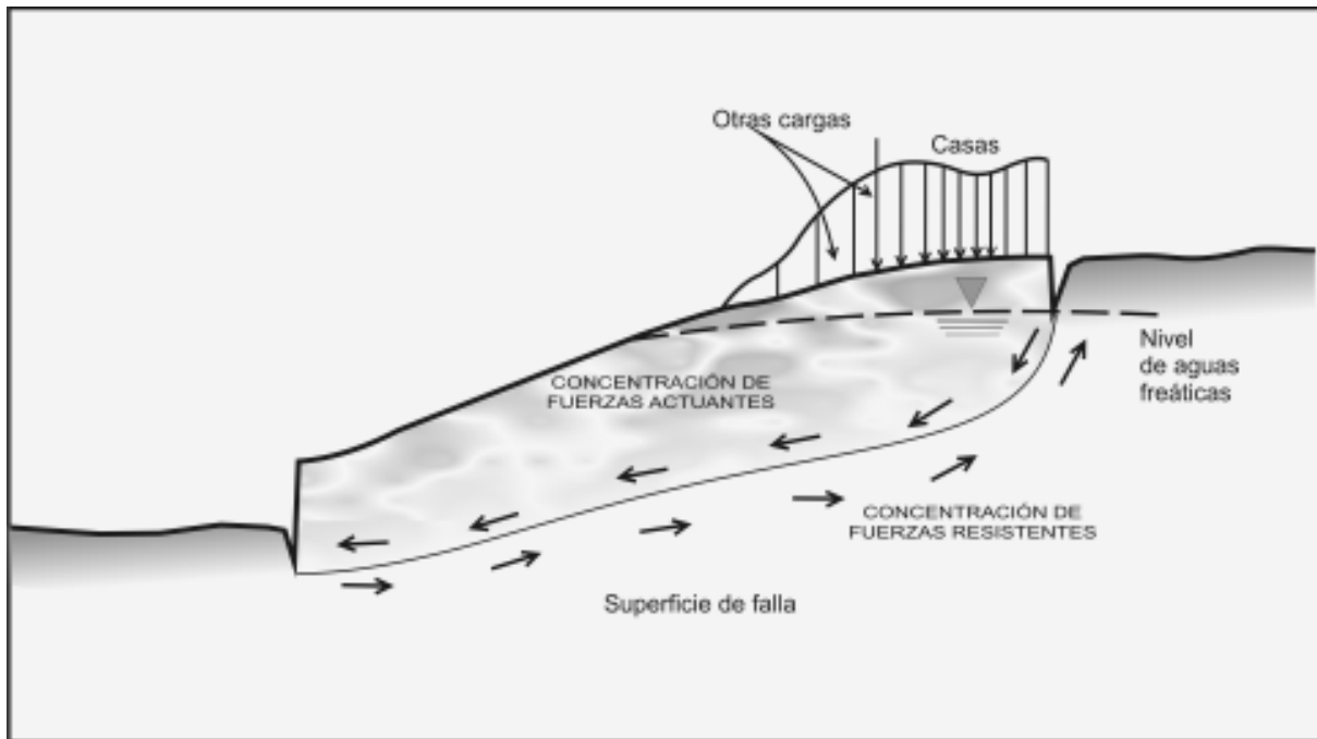
Figura 12. Esquema de factores de inestabilidad
